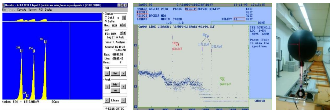
Espectro alfa - Espectro gama - Sala de irradiação do LMRI
